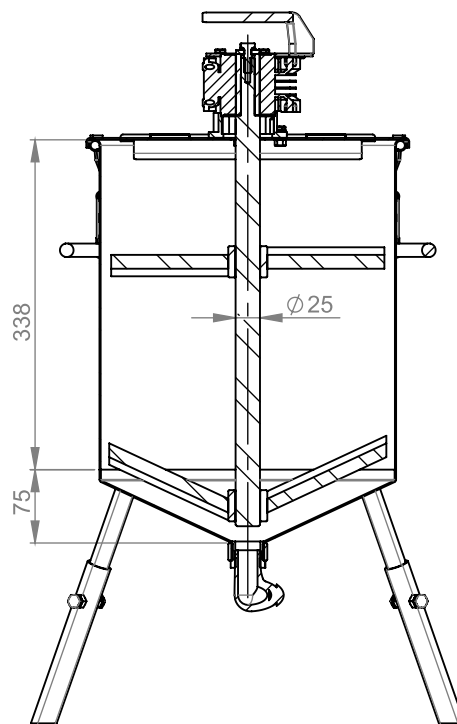
SEZIONE A-A
